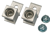
2 PH Main Lug Conversion Kit 150A-225A ECMLK225
