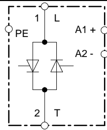
3RF23??-?AA0. 3RF23??-?AA4. Us = 24 V DC
